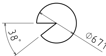
Развертка поверхности
